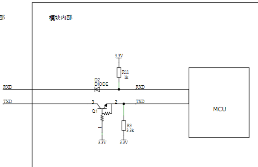
图 5-4 RXD、TXD 引脚内部结构示意图
